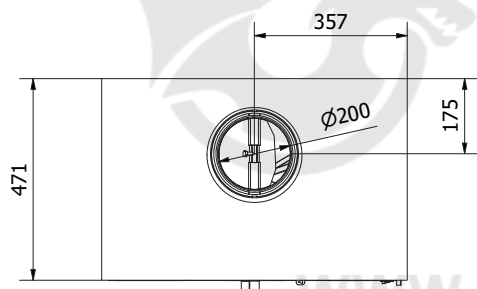
G-G ( 1 : 10 )
