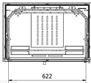
G-G ( 1 : 10 )
