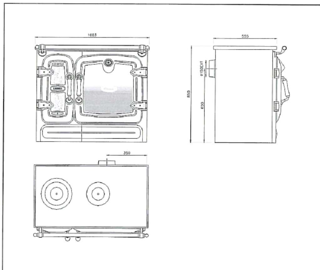
Figura n°3 – Dimensiones en mm Cocina Clásica 8.
