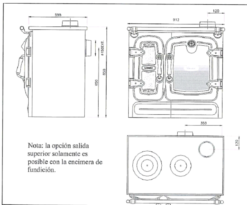
Figura n°2 – Dimensiones en mm Cocina Clásica 7.
