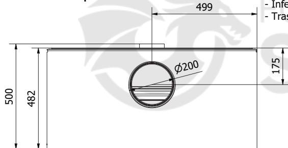
G-G ( 1 : 10 )
