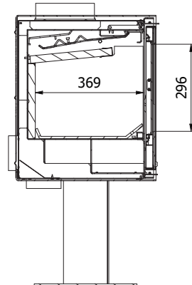
F-F ( 1 : 10 )
