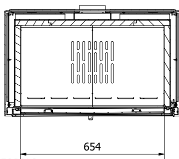
D-D ( 1 : 10 )
