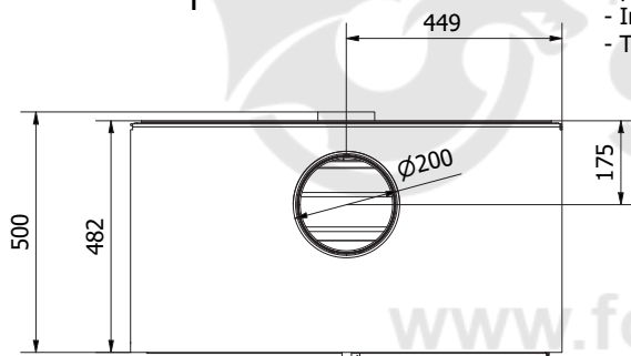
G-G ( 1 : 10 )
