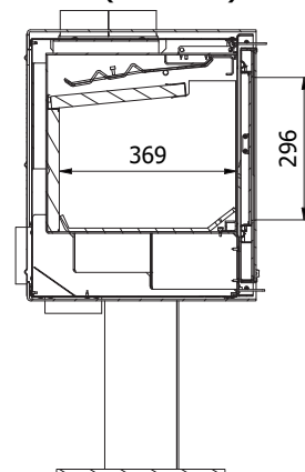
F-F ( 1 : 10 )
