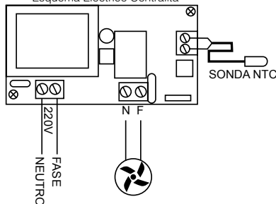
Esquema Eléctrico Centralita
