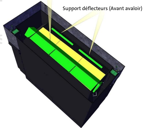
Support déflecteurs (Angle tuyère)
