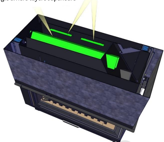
Angle arrière tuyère supérieure
