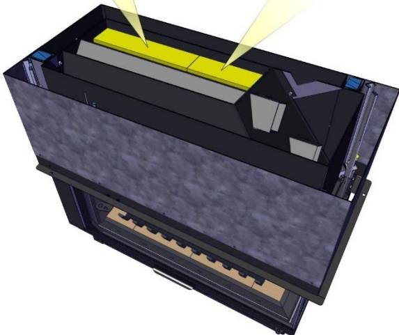
83172 Déflecteur supérieur latéral 258 x 90
