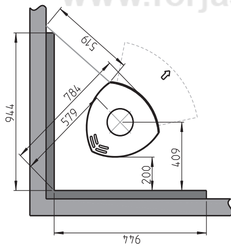
Jötul F 370 Advance - Distancia mínima a una pared de material no combustible
