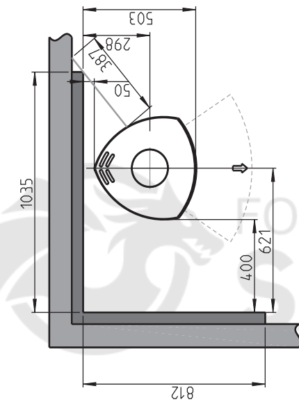
Jötul F 370 Advance - Distancia mínima a una pared de material no combustible
