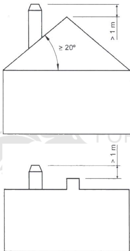
Figura n°4 - Distancias desde el remate hasta la cumbrera del tejado
