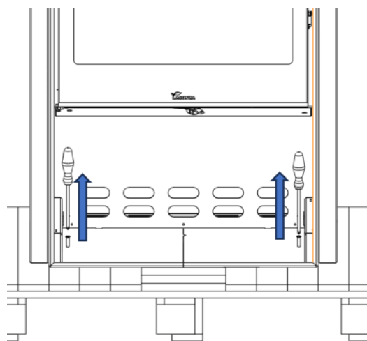
Figura nº3 - Retirada de los tornillos
