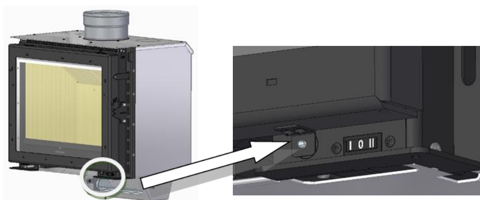
Figura 55 – Ajuste de la manilla de la puerta, funcionamiento del microinterruptor
