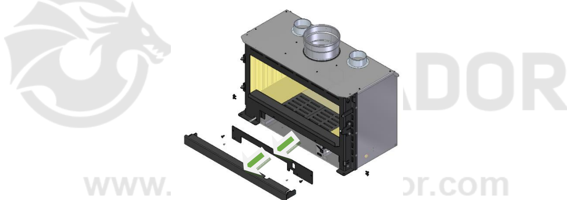
Figura 44 - Desmontaje de la tapa inferior y de la cubierta inferior
