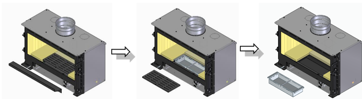
Figura 45 – Retirada de accesorios
