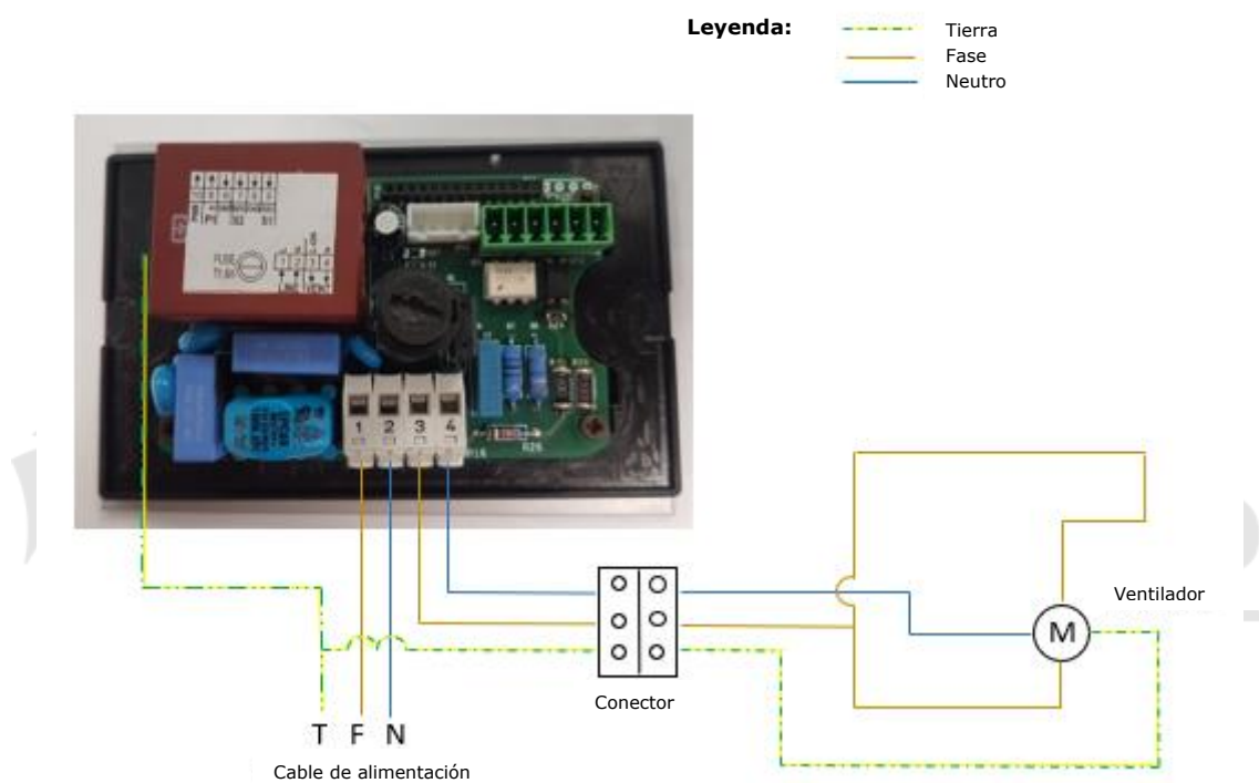
Figura 56 – Esquema eléctrico de la ventilación tangencial
