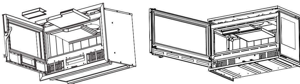
Smontaggio del deflettore su apparecchi PANORMAIC - sx - e GALAXY/TAURUS - dx
