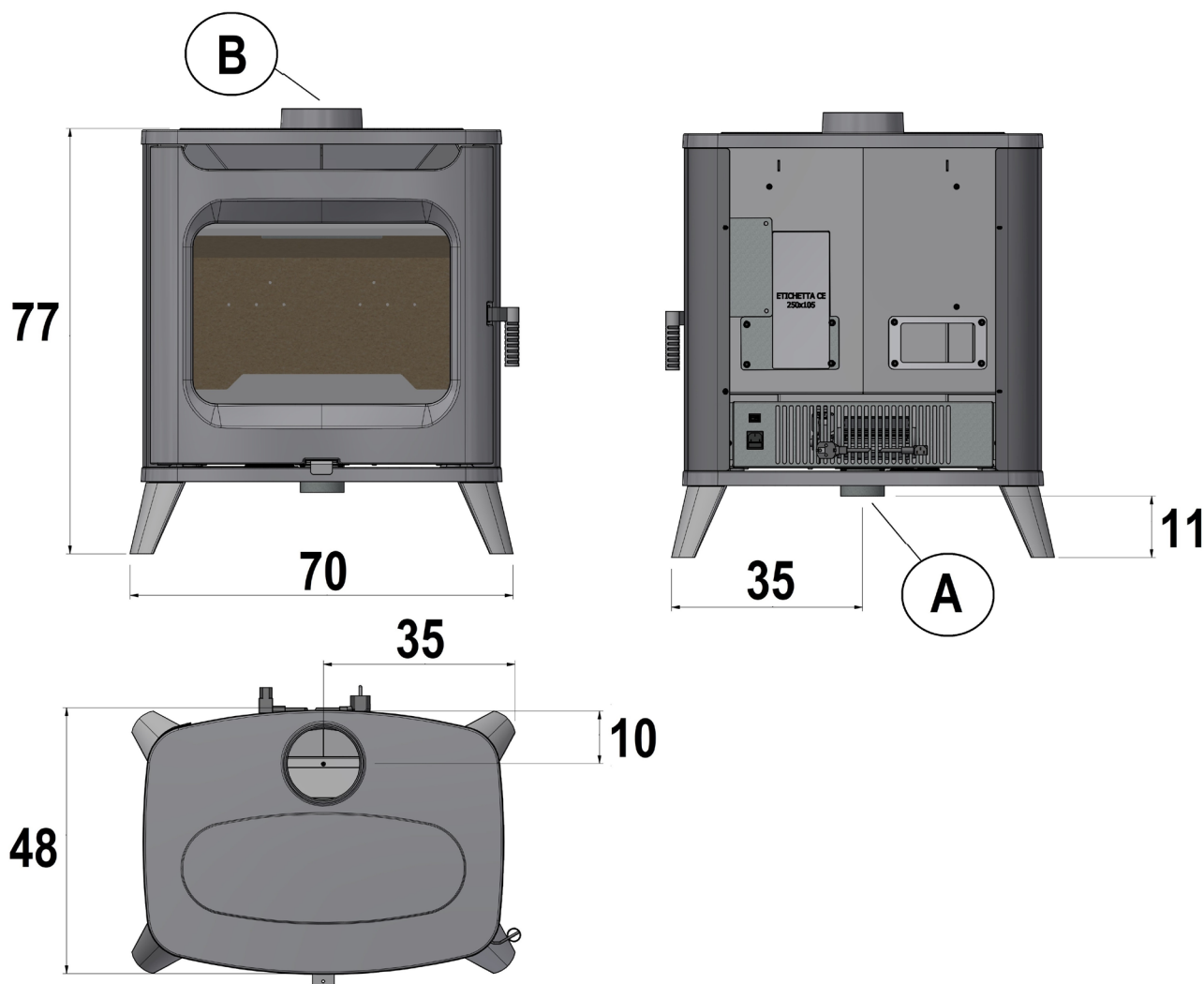
Fig. 11 - Dimensiones generales: HUBLLOT Wood
