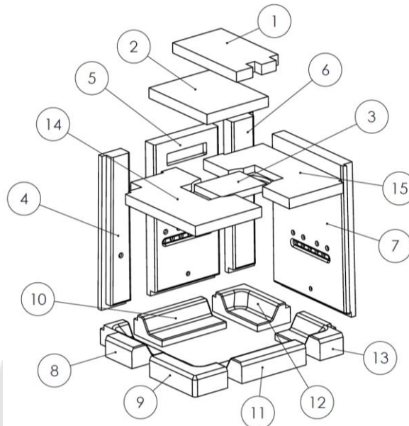
Figura nº47 - Despiece hogar vermi IZARO 60 CLI
