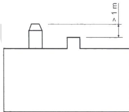
Figura nº23 - Distancias desde el remate hasta la cumbre del tejado
