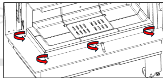
Figura nº15 - Desatornillar los 8 tornillos, 4 superiores y 4 inferiores que amarran el marco exterior
