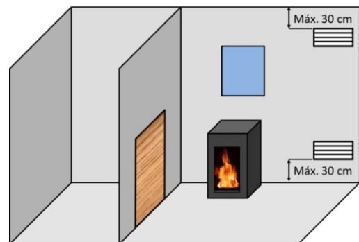
Figura nº4 - Esquema orientativo para rejillas de ventilación
