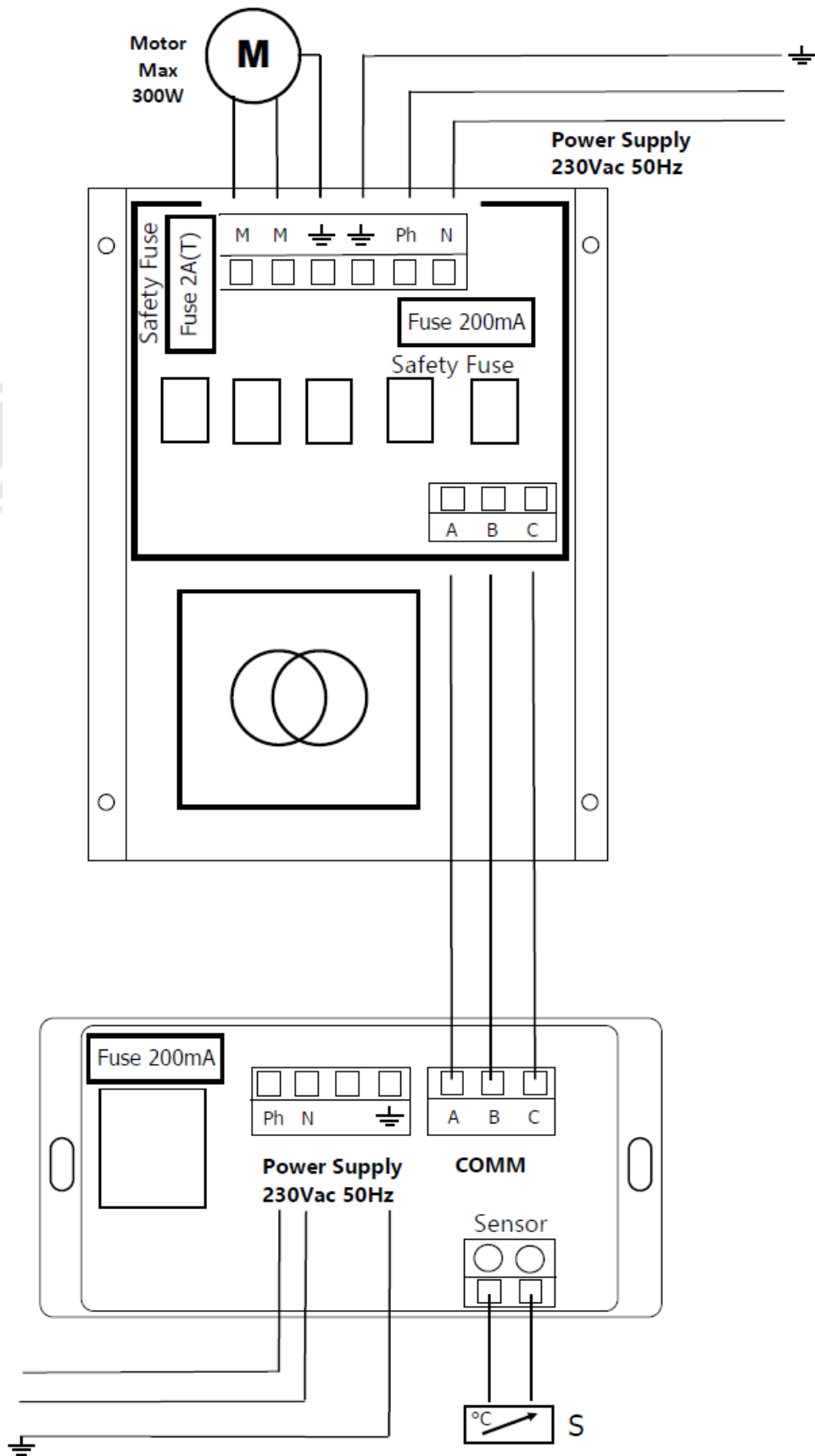
Figura nº18 - Conexiones a realizar en controlador y el módulo de potencia de la Iزارو C/V
