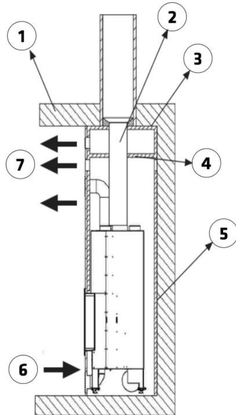
Figura n°7 - Esquema interior del cerramiento
