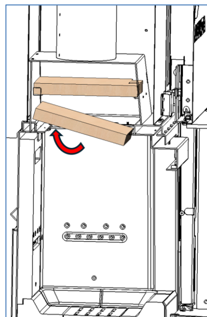
Figura n°34 - Desmontaje del deflector medio Iزارو 60 CLI
