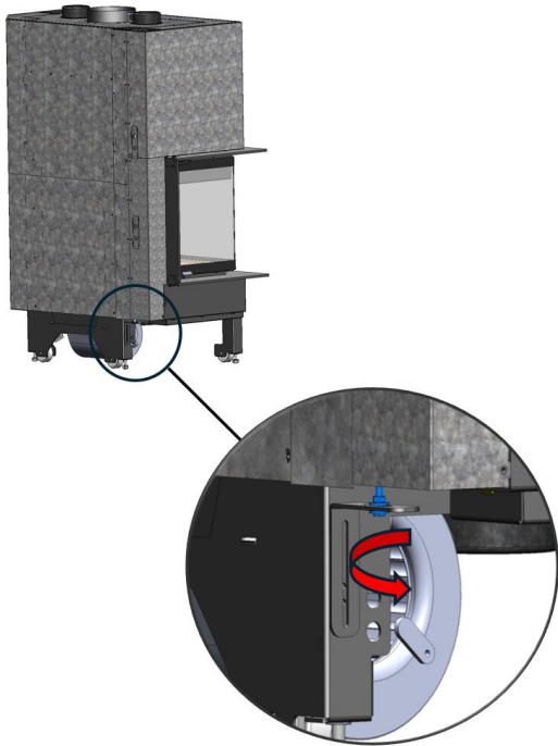
Figura n°5 - Acceso para soltar los tornillos de amarre de los contrapesos IZARO CLI
