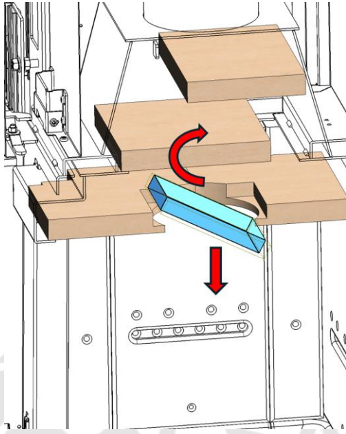
Figura n°31 - Desmontaje catalizador
