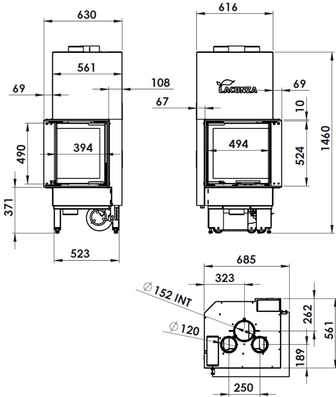
Figura n°2 - Dimensiones en mm del aparato IZARO 60/STAR CLD
