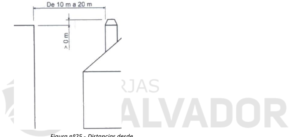
Figura nº25 - Distancias desde el remate hasta objetos entre 10 y 20m
