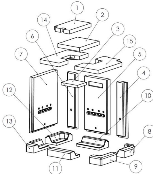
Figura nº49 - Despiece hogar vermi IZARO 60 CLD
