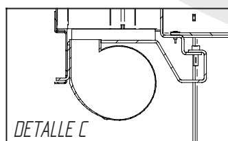
LA TURBINA QUEDA FIJADA A SU SOPORTE POR TRES TORNILLOS.
