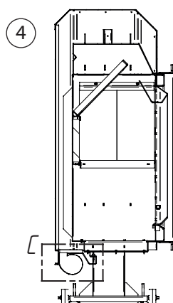
LA TURBINA QUEDA FIJADA A SU SOPORTE POR TRES TORNILLOS.
