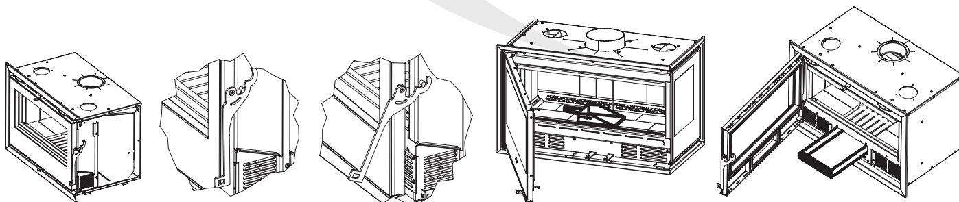
Pala recoge cenizas en PANORAMIC -izq.- y cajón cenicero en GALAXY/TAURUS -dch.-
