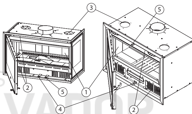
Elementi principali dell'apparecchio: PANORAMIC -sx- e GALAXY/TAURUS -dx-
