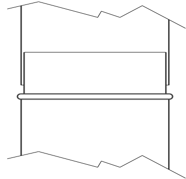
Figura 2. Sentido correcto de los tubos por el exterior de la vivienda, el agua de la lluvia no entra al interior del tubo por los empalmes de los tubos.
