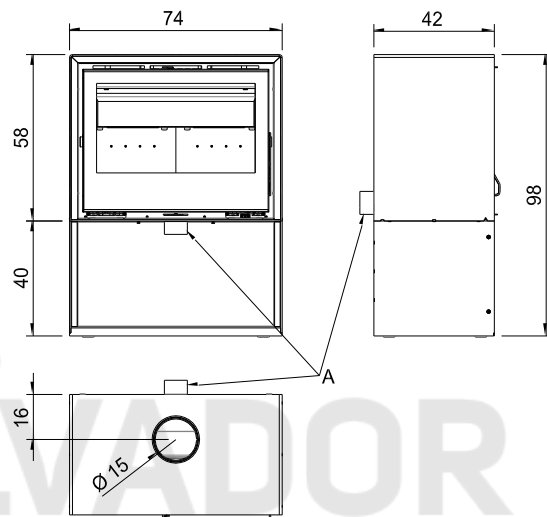
RI 70 con Leñera/ RI 70 with Log box.
