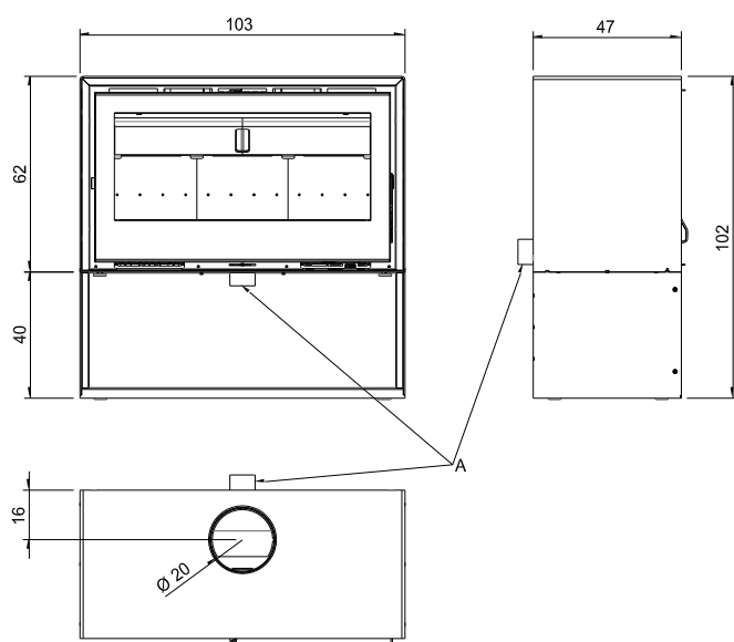
RI 100 con Leñera/ RI 100 with Log box.
