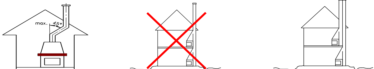
Figura 20 - Instalación de conductos y chimeneas
