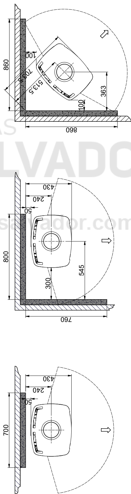
Distancia mínima a una pared de material combustible protegida con cortafuegos (con ventanas laterales)
