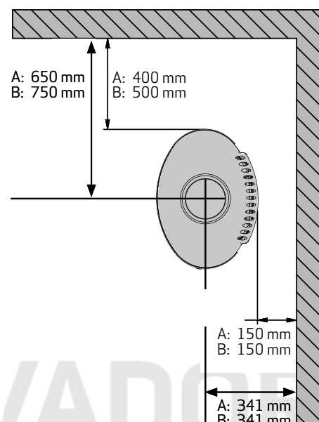
Instalación paralela a la pared posterior
