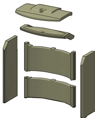
Revestimiento de la cámara de combustión
