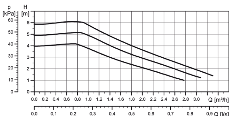
Gráfico del caudal (Q) / altura de elevación (H)
