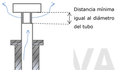
Figura 28 - Unión correcta
