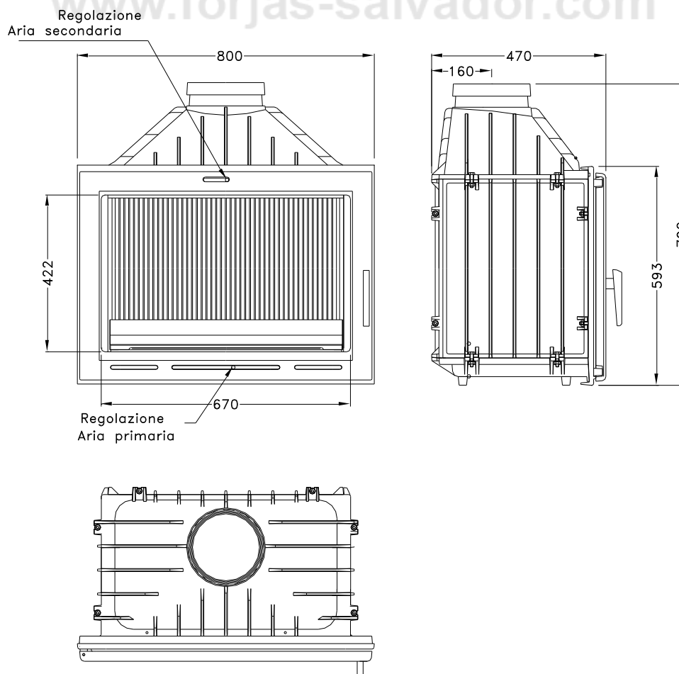
Fig. 17 Dimensioni H-03-80
