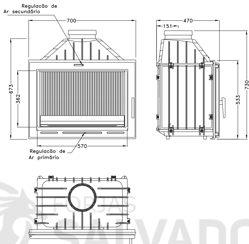
Fig. 16 Dimensões EQR-70
