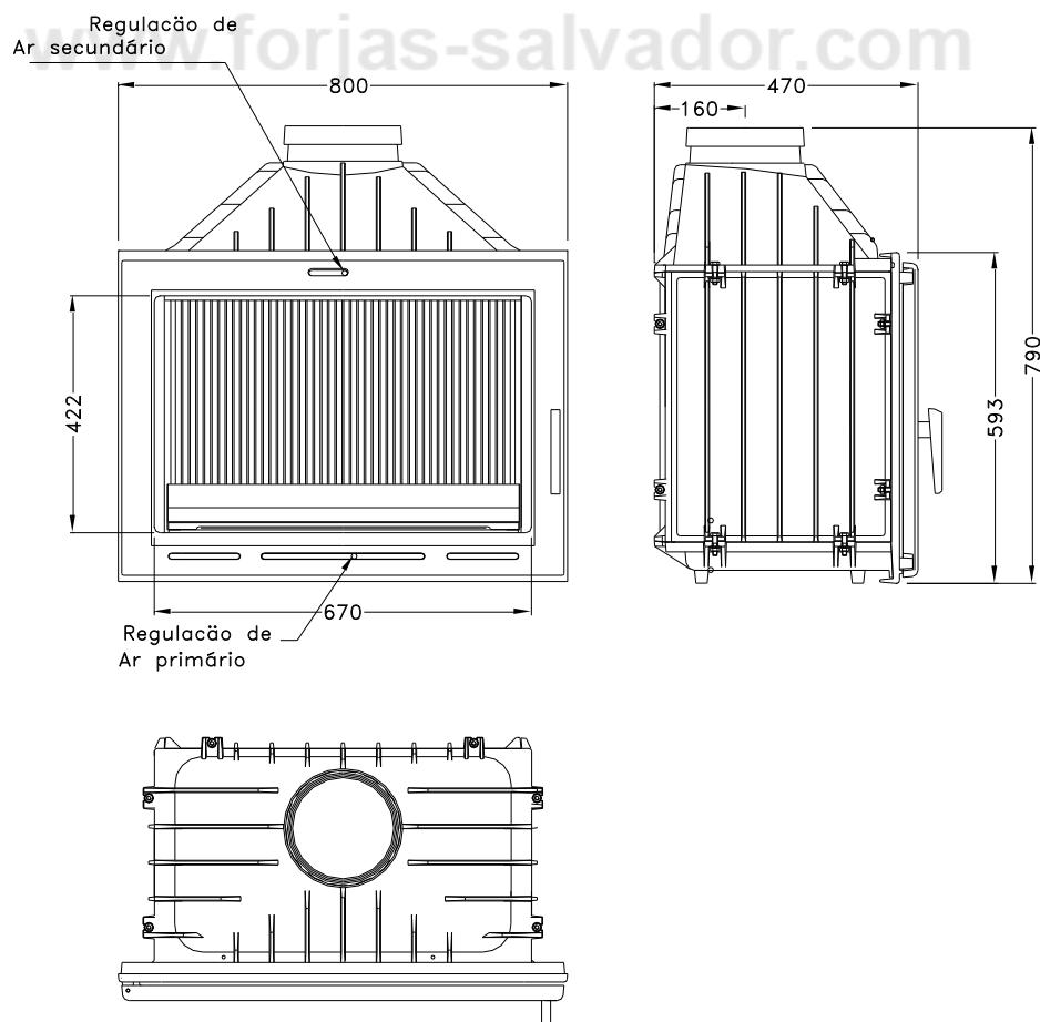
Fig. 17 Dimensões EQR-80
