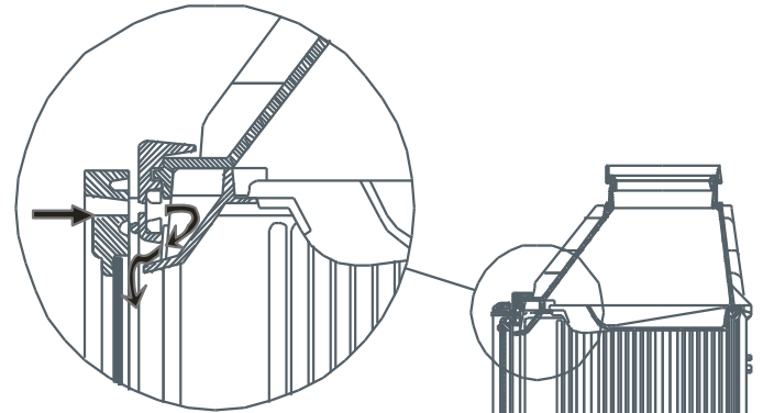
Σχ.-12 Λεπτομέρεια παροχής δευτερογενή αέρα
