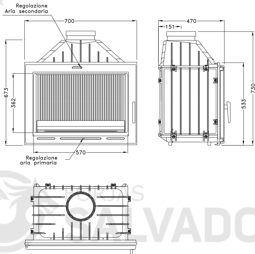
Fig. 16 Dimensioni H-03-70
